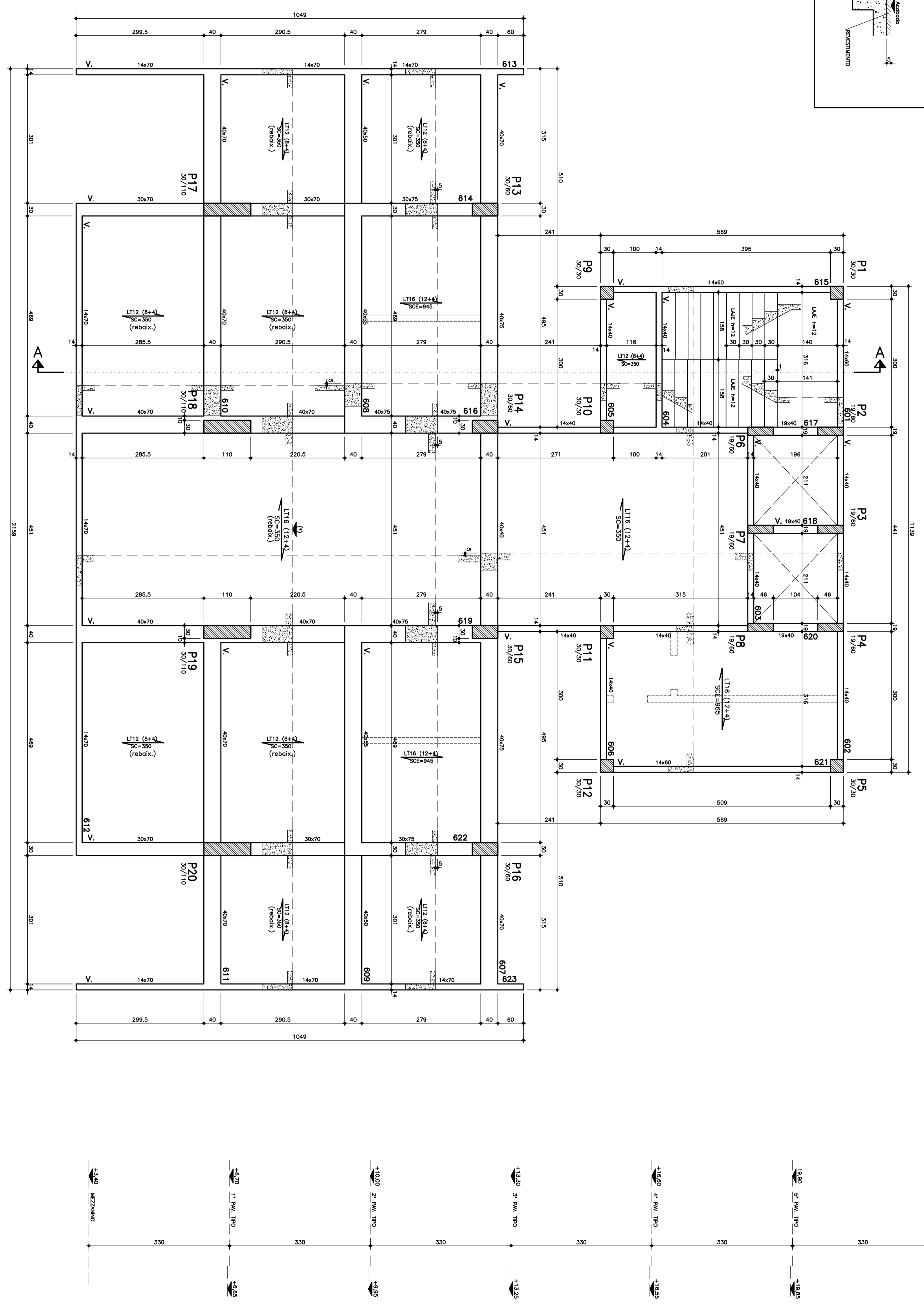
PAVIMENTO TIPO 1º AO 3º (3x) ESCALA 1:50
