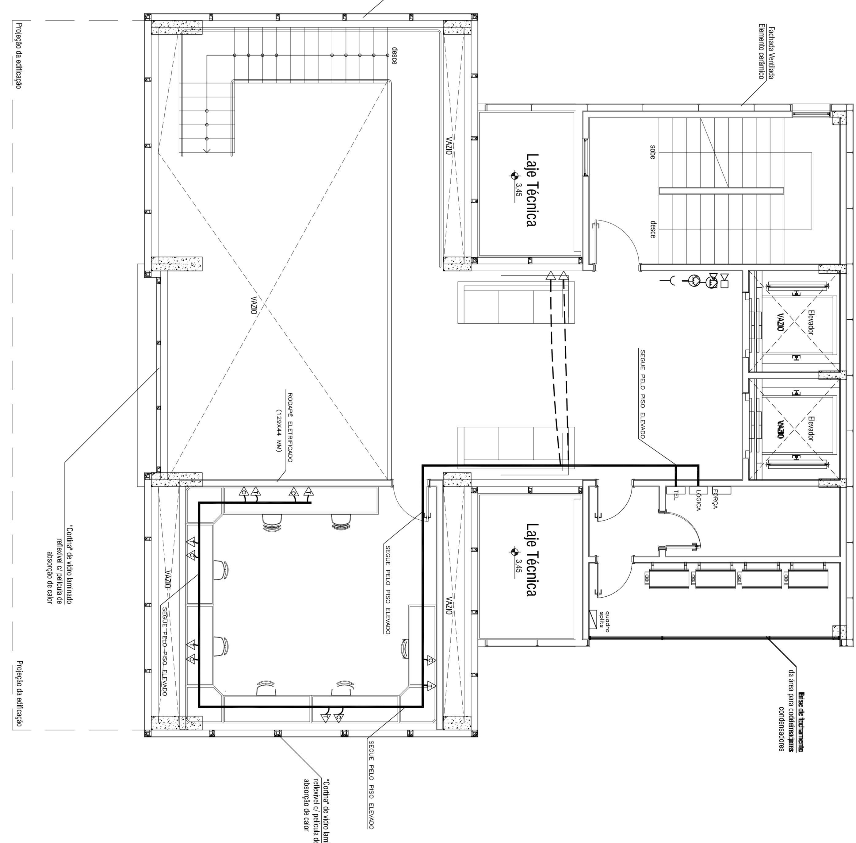
MEZANINO ESCALA 1:50
